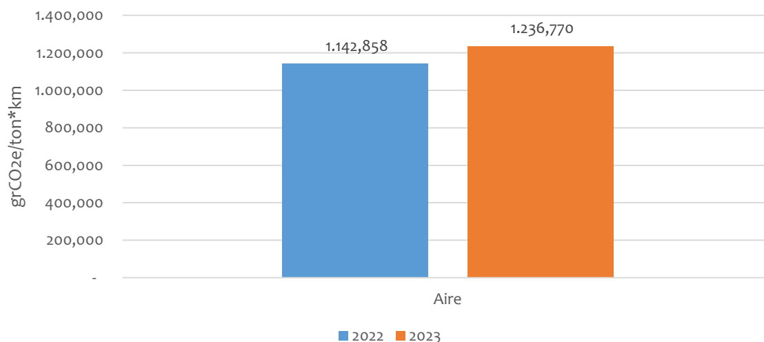
Gráfica 8. Comparativo emisiones específicas transporte de aire
