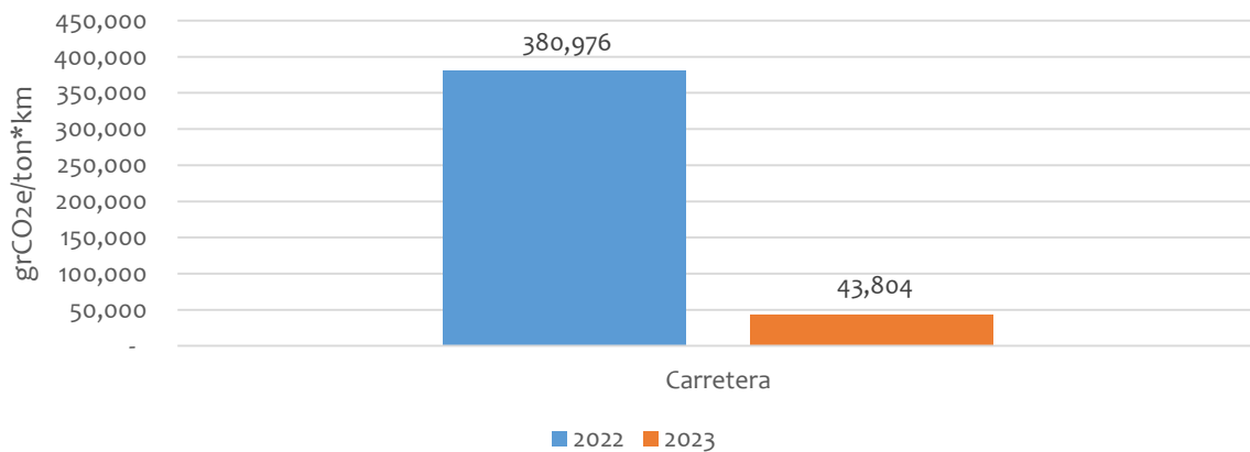
Gráfica 7. Comparativo emisiones específicas transporte de carretera
