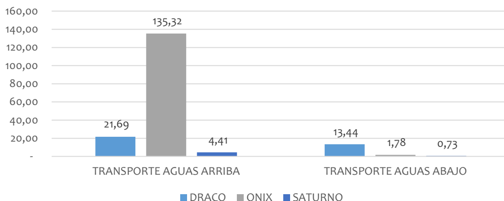
Gráfica 5. Comparativa transportes
